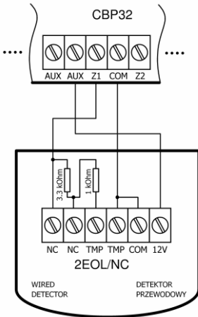
Schemat 2. Łączenie detektorów przewodowych do centrali CBP32 z funkcją alarmu włamaniewego oraz antysabotażowego otwarcia obudowy, zwarcia lub odcięcia linii przewodowej.
