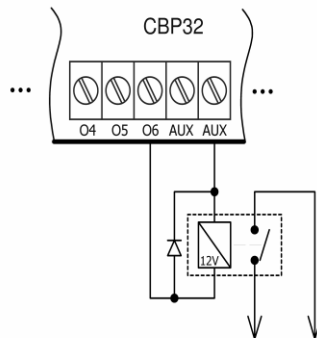
Schemat 5. Łączenie przekaźnika do sterowania urządzeniami zewnętrznymi z wyjść O1-O6 Connection of relay for external devices control via outputs O1-O6
